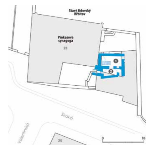
Odkryté konstrukce pozdně středověkých zdí objektu s rituální lázní: 1 – místnost s vodní nádrží; 2 – místnost s otopným zařízením. Podle Michala Trymla, archiv Národního památkového ústavu, územní odborné pracoviště v Praze
